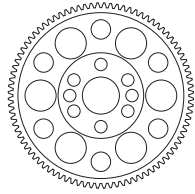
大齒盤 88T-48P ×1 Spur gear 88T-48P 210013
