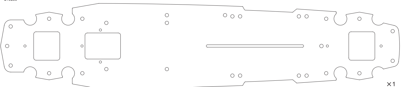
碳纖維底盤 (SSG) Carbon lower deck (SSG) 210250
